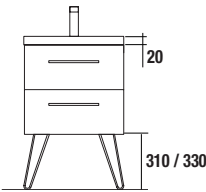
PÉS COM ALTURA 330 mm PARA UTILIZAR COM LAVATÓRIO INTEGRAL
